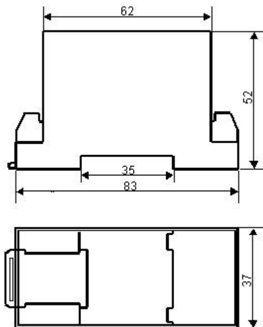
图 4.2、产品尺寸图
